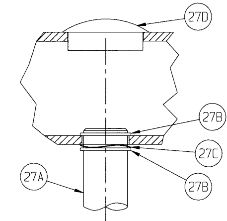
GUIDE ROD DETAIL
